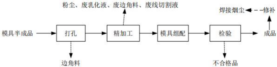
图 2-3 塑料模具生产工艺
