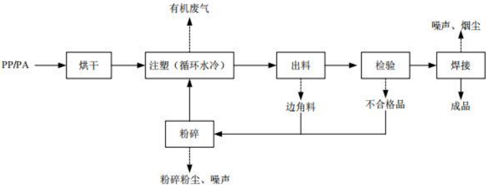
图 2-5 汽车用塑料件生产工艺
