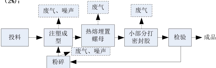
图 2-2 汽车用塑料件生产工艺流程和产污环节图
