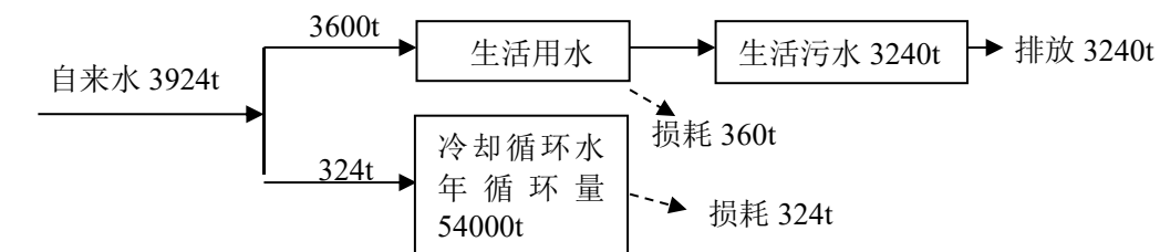
图 2-1 本项目实施后水平衡图
