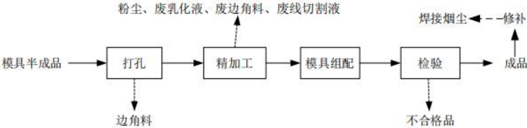
图 2-4 塑料模具工艺流程图
